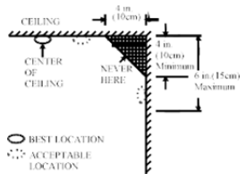
Figure 4: Beste und akzeptable Montageorte für Melder
